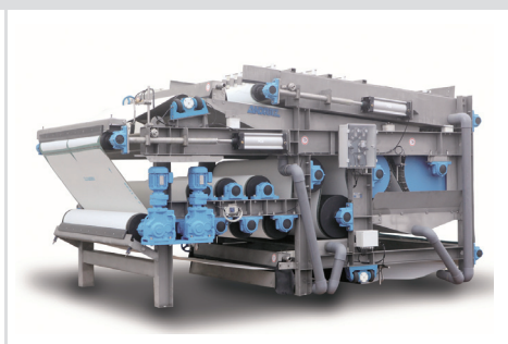
Belt press Siebbandpresse
