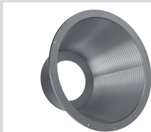
Centrifuge insert basket for solid / liquid separation Zentrifugenkorb für die Fest-Flüssig-Trennung
