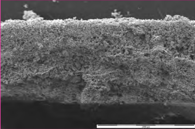
Abb. 4: Querschnitt versinterter Filterkuchen
