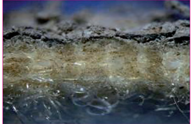
Abb. 6: Filtermedienquerschnitt mit Staubabscheidung auf der Oberfläche und partikelfreie Tiefenfasern
